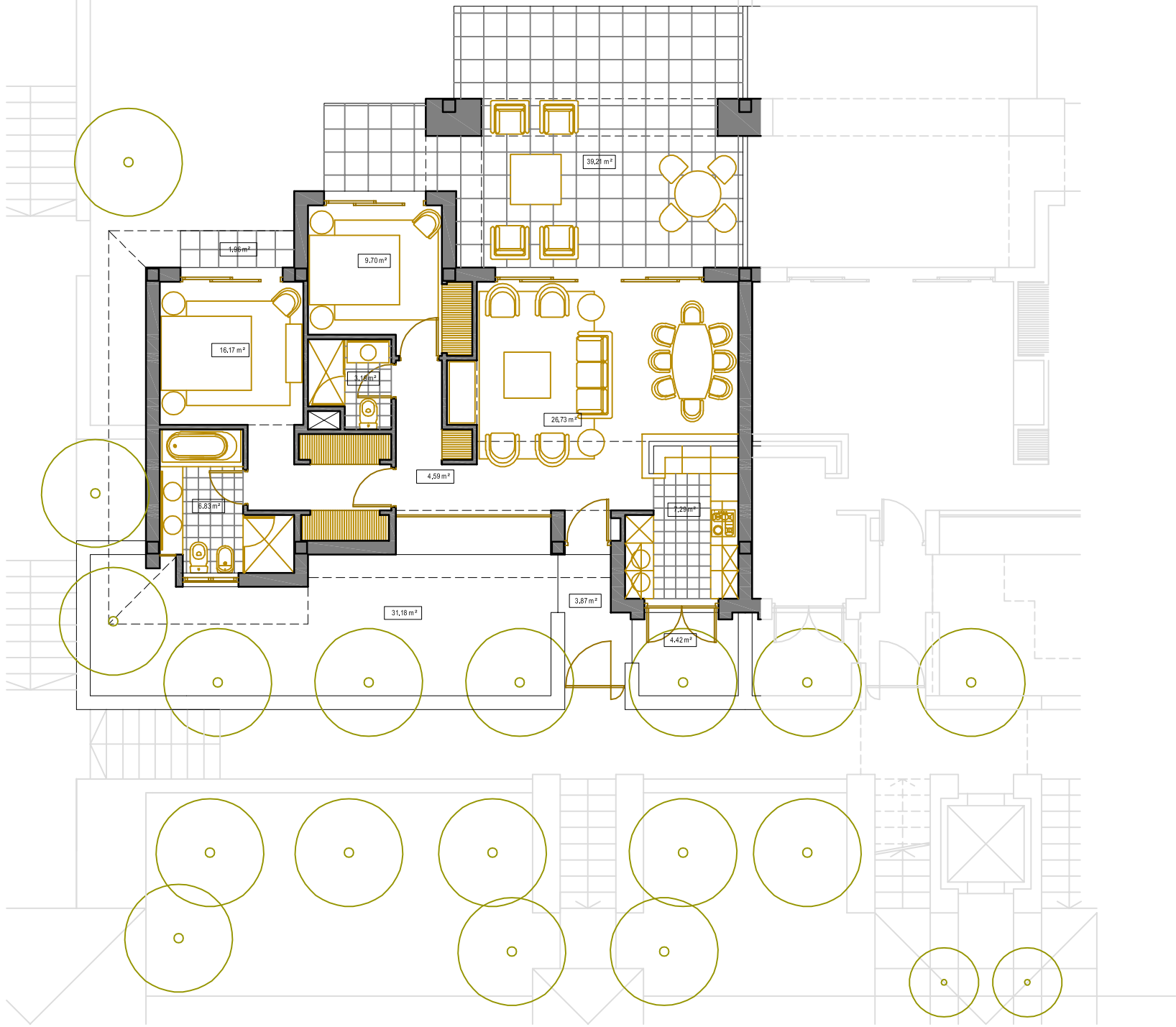
VIVIENDA 31 TIPO A PLANTA BAJA BLOQUE 3
